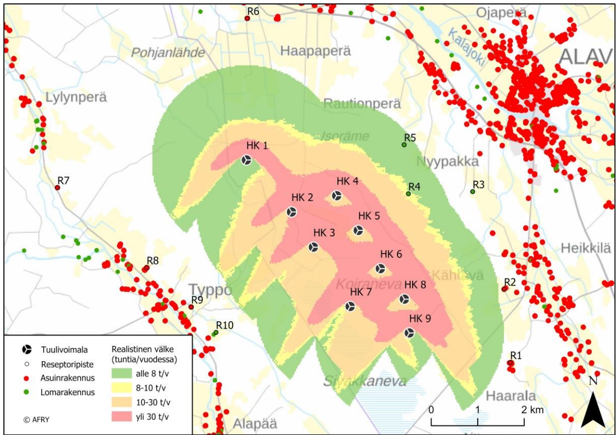
Kuva 12-28. Välikkeen realistinen määrä tunteina vuodessa (aurionpaistehavainnot otettu huomioon) Hangaskurunkankaan yhdeksän voimalan sijoitus suunnitelmalla. Mallinnus on tehty tuulivoimaloilla, joiden napakorkeus on 200 m ja roottorin halkaisija 200 m.
