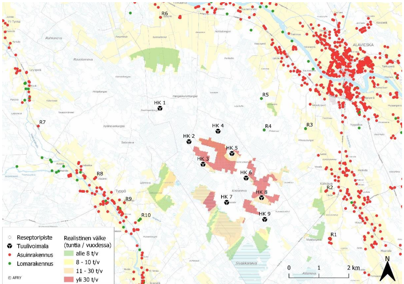
Kuva 12-30. Välikkeen realistinen määrä tunteina vuodessa (auringonpaistehavainnot on huomioitu) Hangaskurunkankaan yhdeksän voimalan sijoitussuunnitelmalla, kun puuston vähentävä vaikutus on huomioitu. Mallinnus on tehty tuulivoimaloilla, joiden napakorkeus on 200 m ja roottorin halkaisija 200 m.
