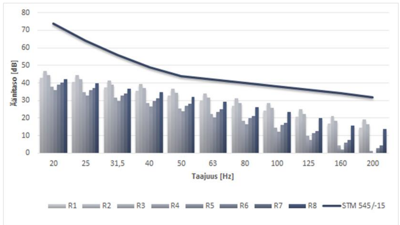
Kuva 12-25. Pientaajuisen melun laskentatulokset lähimmissä reseptoripisteissä R1-R8 taajuualueittain. Sisätilan toimenpiderajat on esitetty mustalla viivalla.
