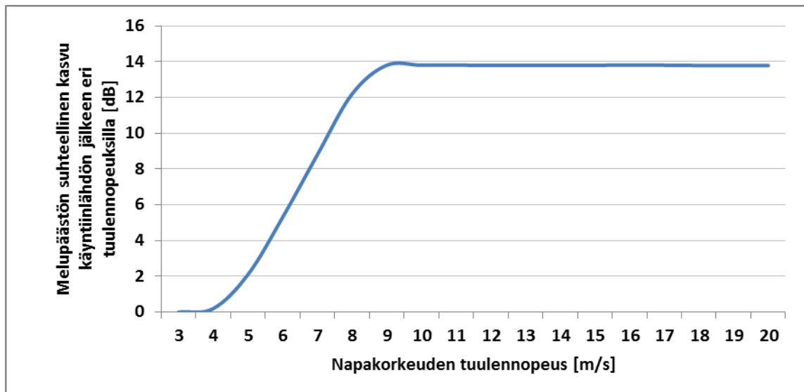
Kuva 12-23. Esimerkkikuva äänipäästön kasvusta napakorkeuden tuulennopeuden mukaan. Äänitason nousu tasoittuu noin 10 m/s tuulisuuden jälkeen.
