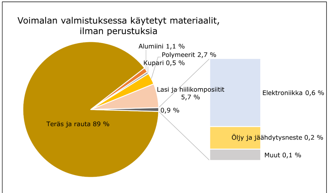
Kuva 12-39. Esimerkki voimalan valmistuksessa käytettävistä materiaaleista pois lukien voimalaperustukset, ja niiden osuus koko voimalan massasta. Voimalamalli: Vestas V150-4,2 MW. (Vestas 2022b)
