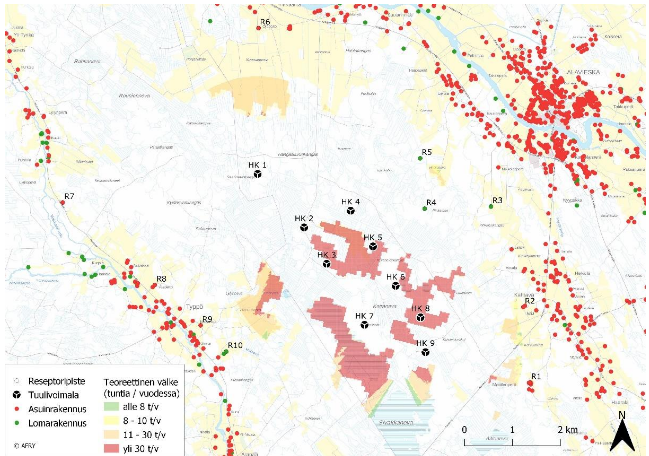
Kuva 12-29. Välkkeen teoreettinen määrä tunteina vuodessa (auringonpaistehavaintoja ei ole huomioitu) Hangaskurunkaan yhdeksän voimalan sijoitussuunnitelmalla, kun puuston vähentävä vaikutus on huomioitu. Mallinnus on tehty tuulivoimaloilla, joiden napakorkeus on 200 m ja roottorin halkaisija 200 m.
