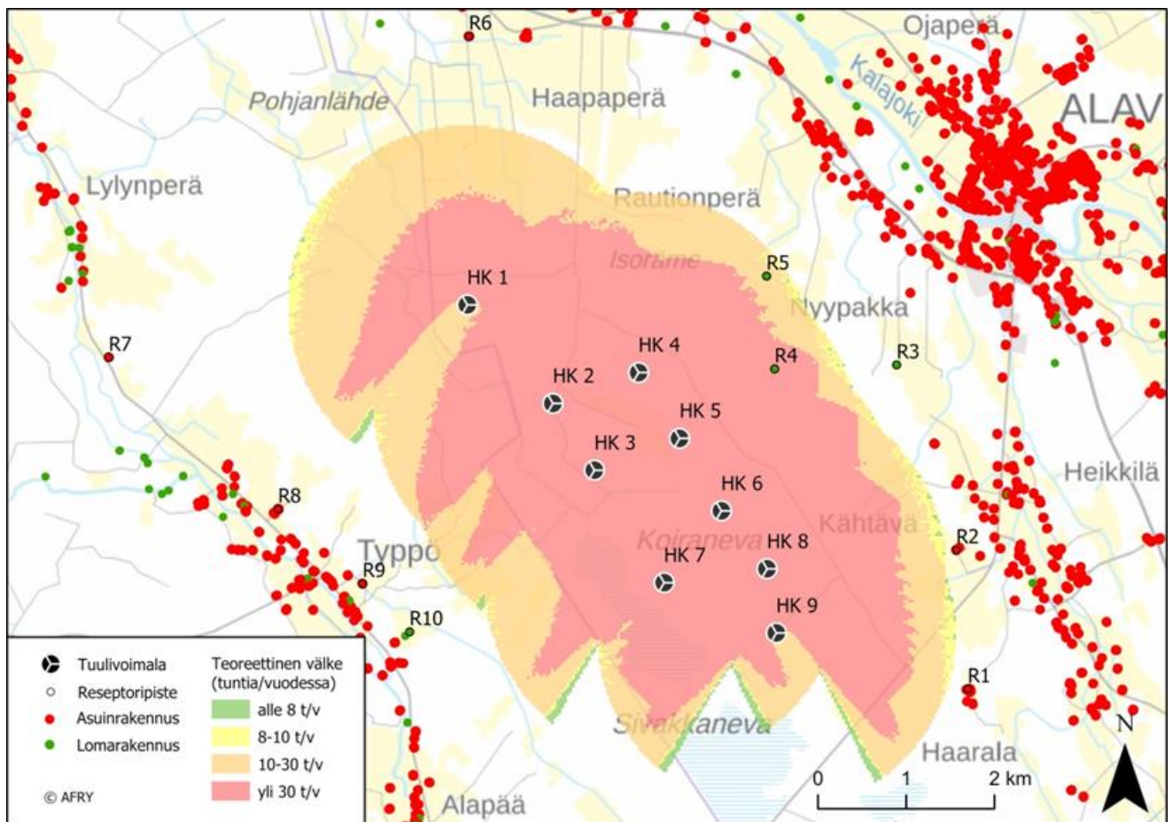
Kuva 12-27. Välkkeen teoreettinen määrä tunteina vuodessa (auriongonpaistehavaintoja ei ole huomioitu) Hangaskurun- kankaan yhdeksän voimalan sijoitussuunnitelmalla. Mallinnus on tehty tuulivoimaloilla, joiden napakorkeus on 200 m ja roottorin halkaisija 200 m.
