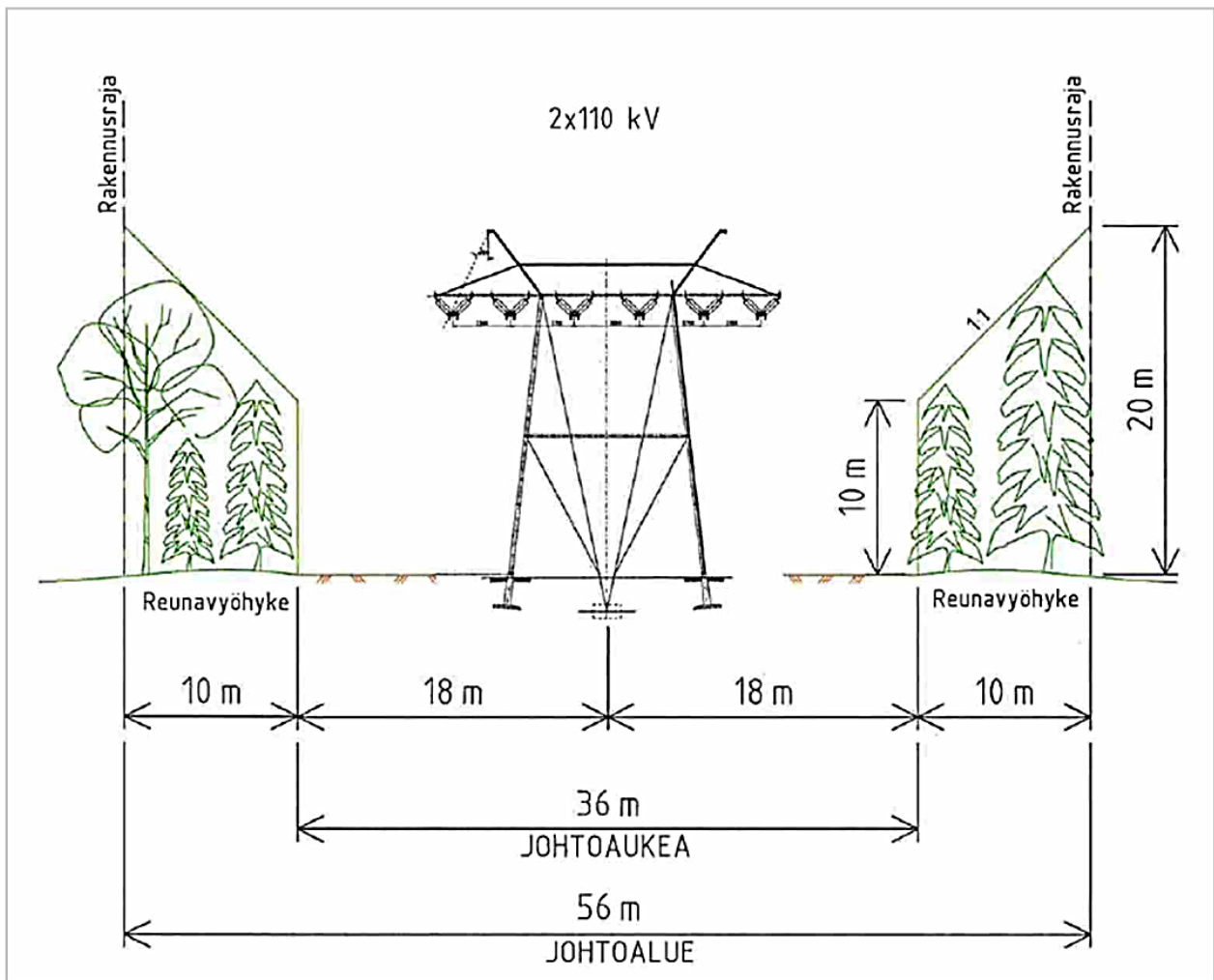
Kuva 7-3. Periaatekuva voimajohdosta, johon tuulipuisto liitetään (Ramboll 2013).
