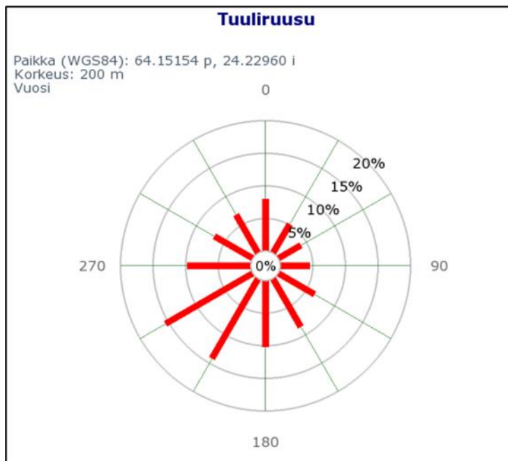
Kuva 9-25. Tuulensuunta hankealueella 200 metrin korkeudella. (Tuuliatlas 202)
