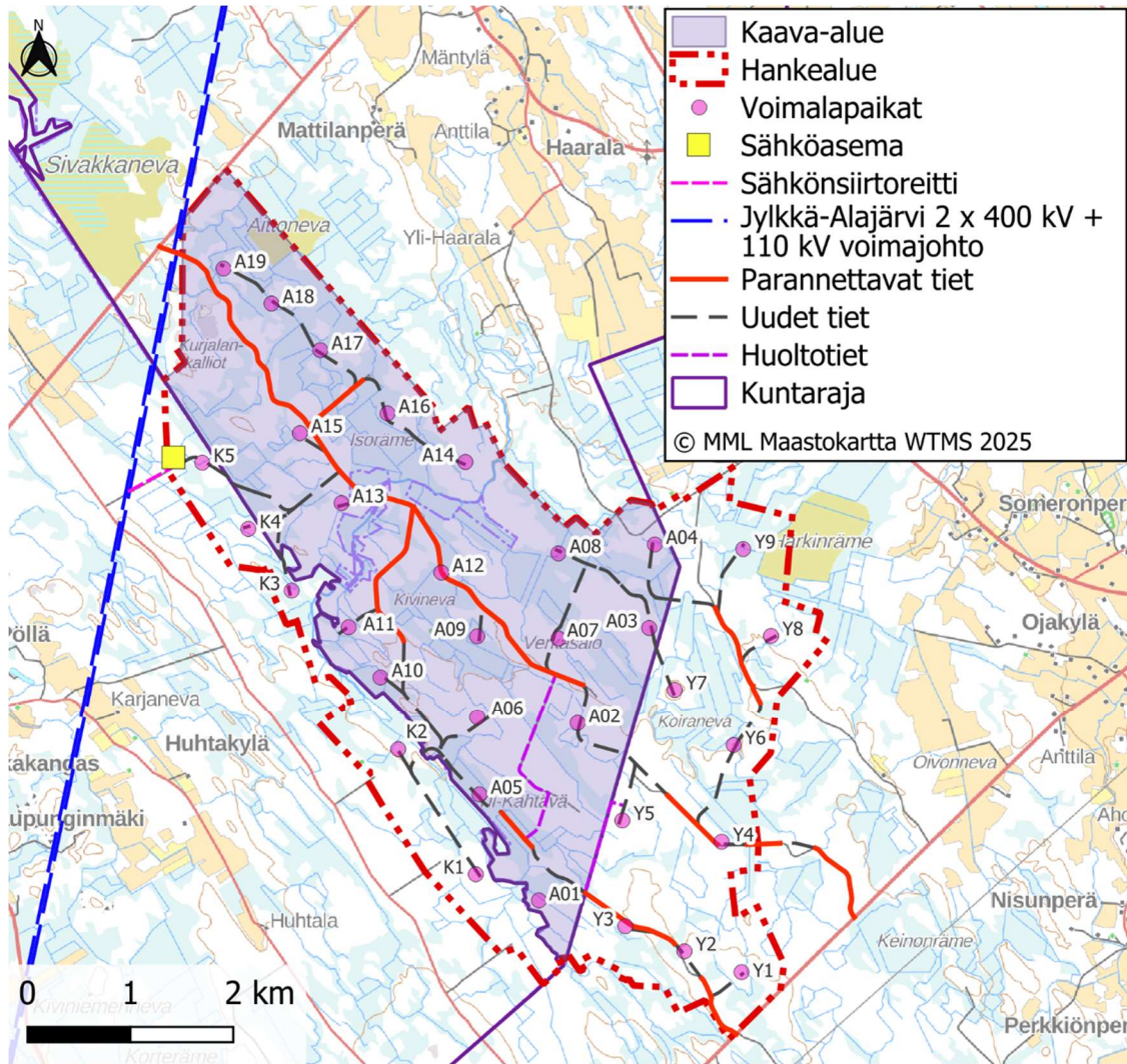
Kuva 4. Verkasalon tuulivoimapuiston tuulivoimaloiden tarkentunut sijoittelu hankealueella. Alavieskan kaava-alue korostettu sinisellä värillä.
