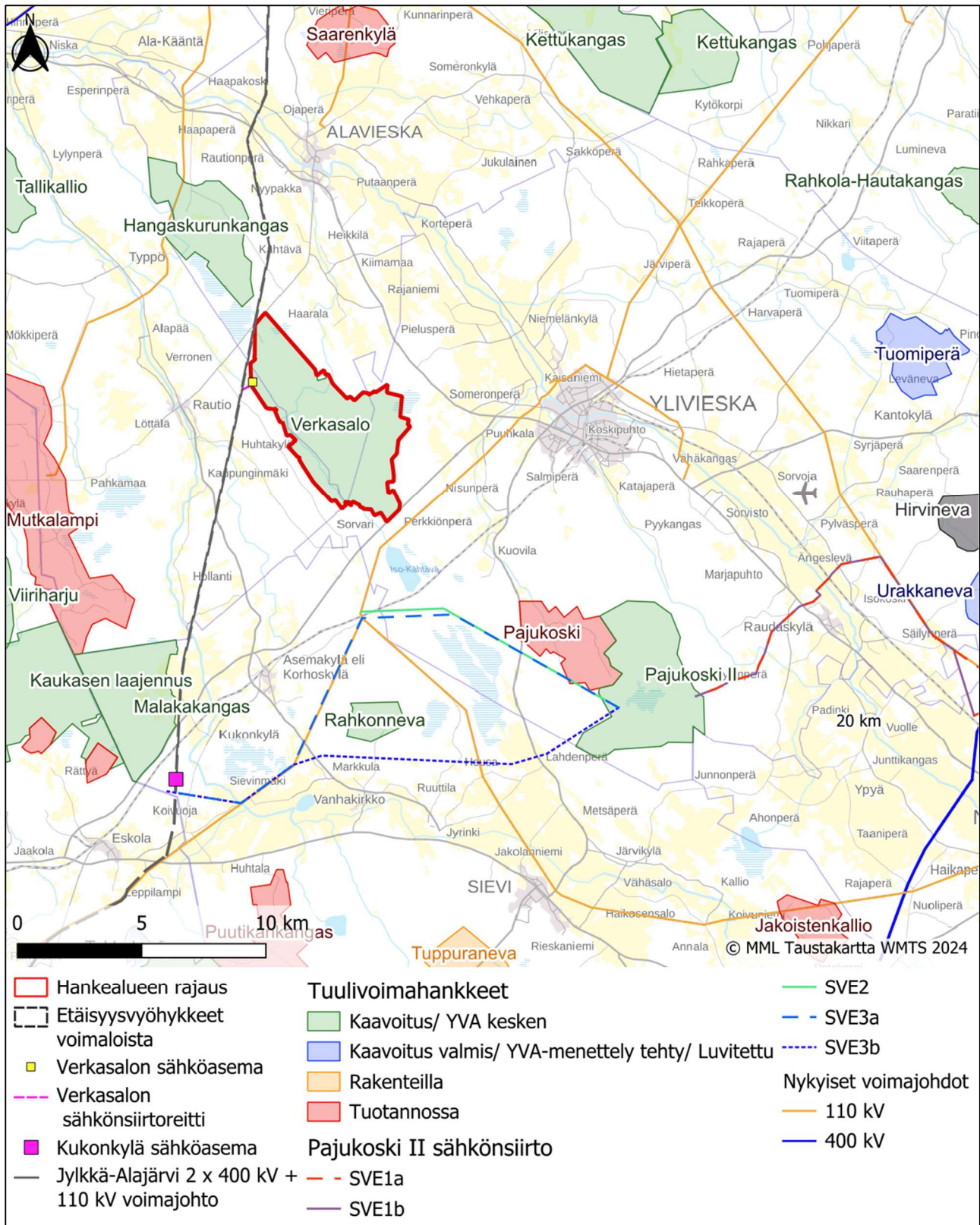
Kuva 61. Verkasalon sähkönsiirto, Fingridin Jylkkä-Alajärvi-linja (Lakeuslinja) sekä Pajukoski II:n ja Hangaskurunkankaan sähkönsiirtoreitit.
