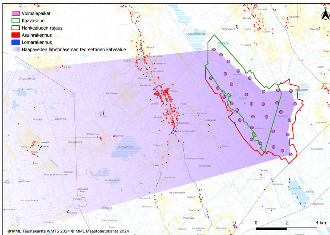
Kuva 56. Verkasalon tuulivoimalat voivat häiritä antenni-tv-vastaanottoa alueella, jossa tuulivoimalat sijoittuvat Haapaveden lähettinasemalta tulevan signaalin ja tv-vastaanottimen väliin. Kaava-alue on korostettu vihreällä rajalla.
