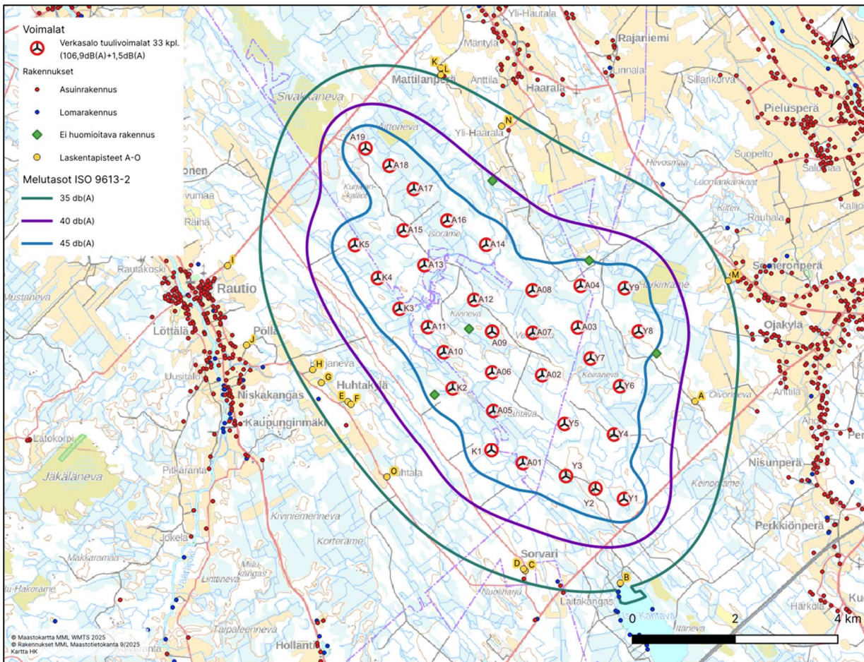
Kuva 48. Melumallinnustulos Verkasalon kaavavyöksymisvaiheen voimalasijoittelun mukaan. Tuulivoimaloiden napakorkeutena on käytetty 232,5 metriä. Voimaloiden A17, A18 ja A19 napakorkeutena on käytetty 192,5 metriä. Voimaloiden lähtömelutaso on 106,9 dB ja siihen on lisätty 1,5 dB varmuusarvo. Karttaan on merkitty laskentapisteinä käytetyt lähimmät asuin- ja lomarakennukset kirjaimilla A–O.
